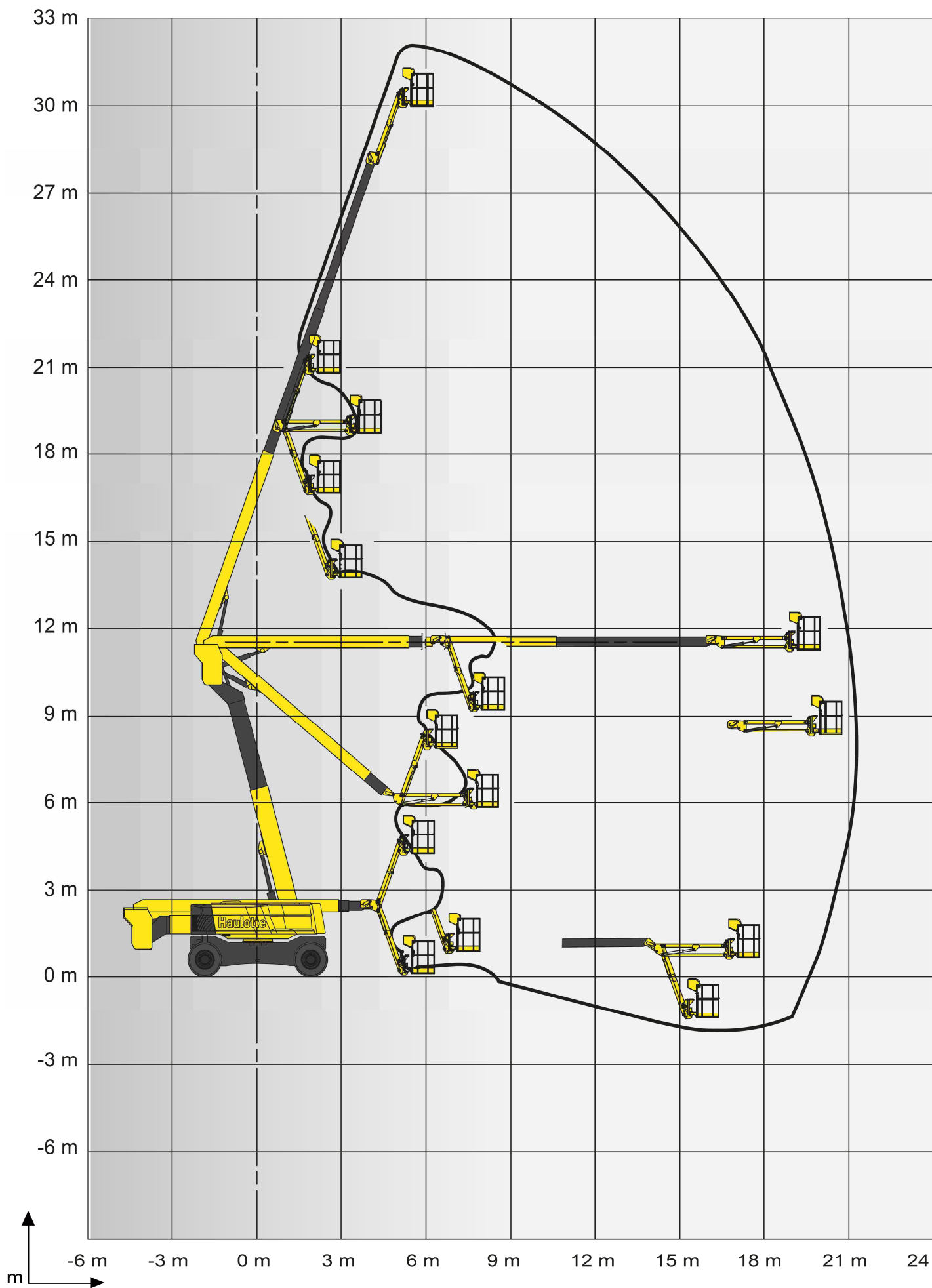
JLG 1350SJP
